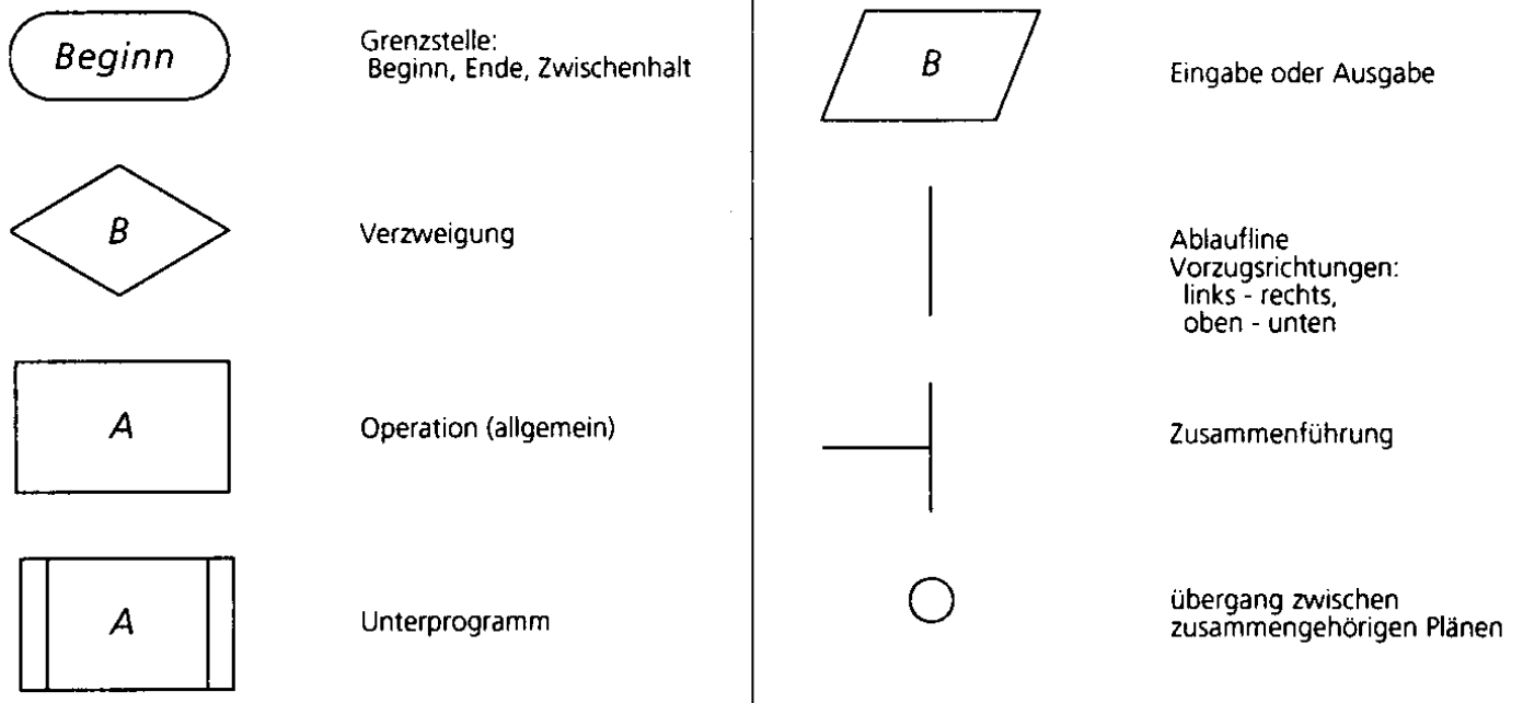
Abbildung 11.5: Symbole für Programmablaufpläne nach DIN 66 001
